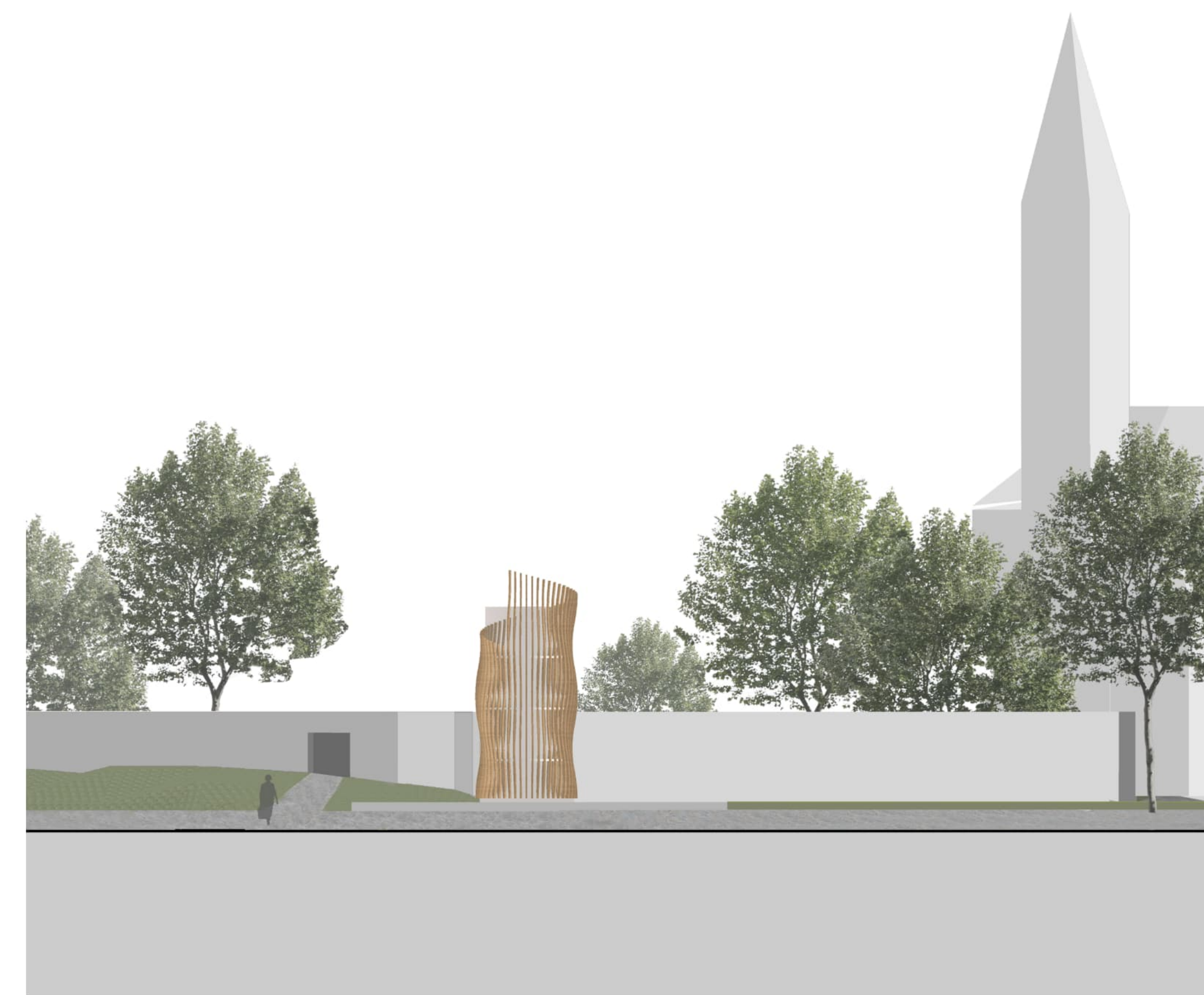
Ansicht Nordwest Lüftungsturm 1:200
