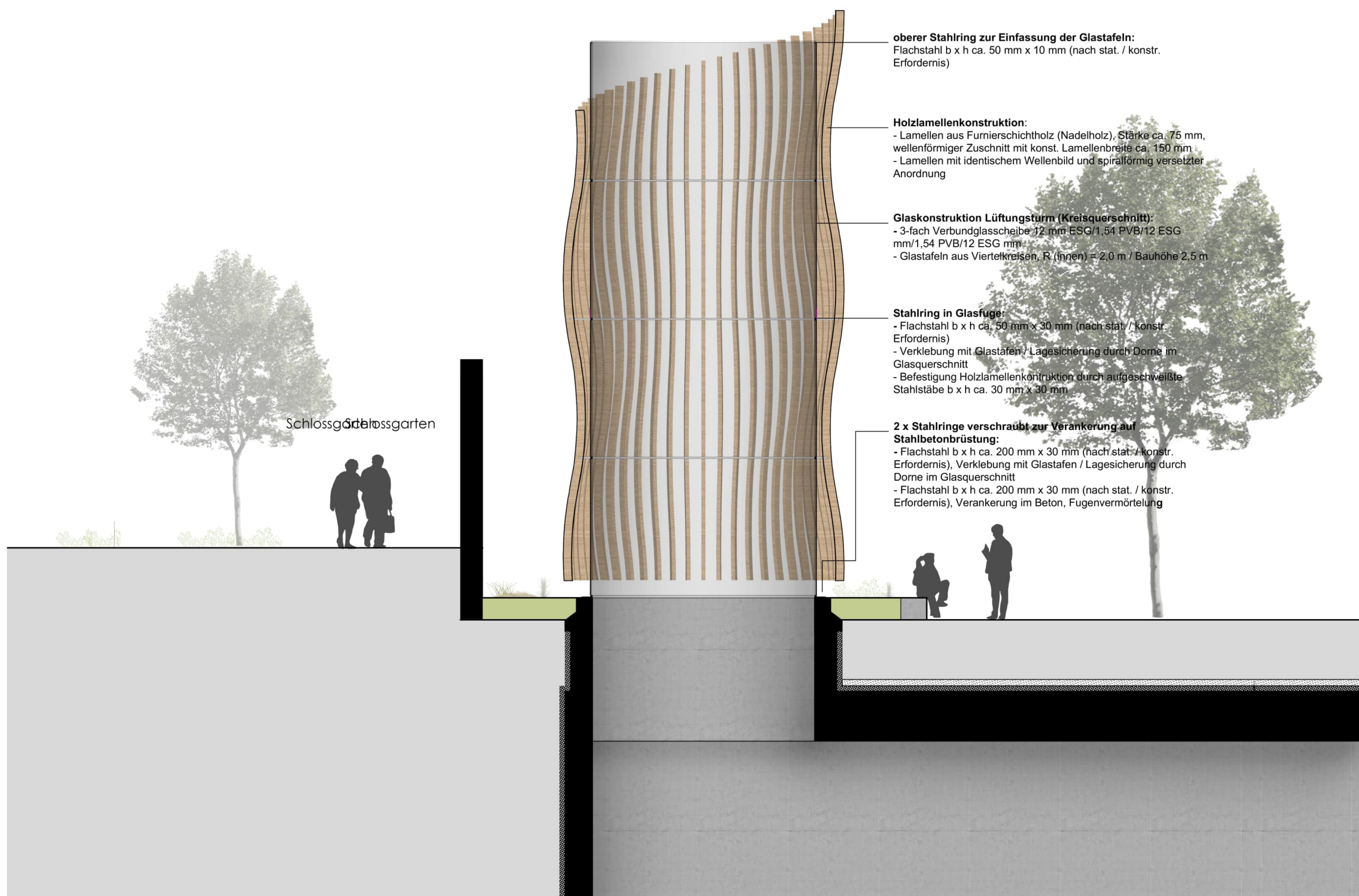
Detailschnitt Lüftungsturm 1:50
