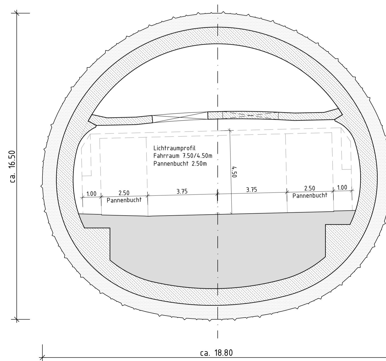
Tunnelquerschnitt Pannenbucht M 1:100
